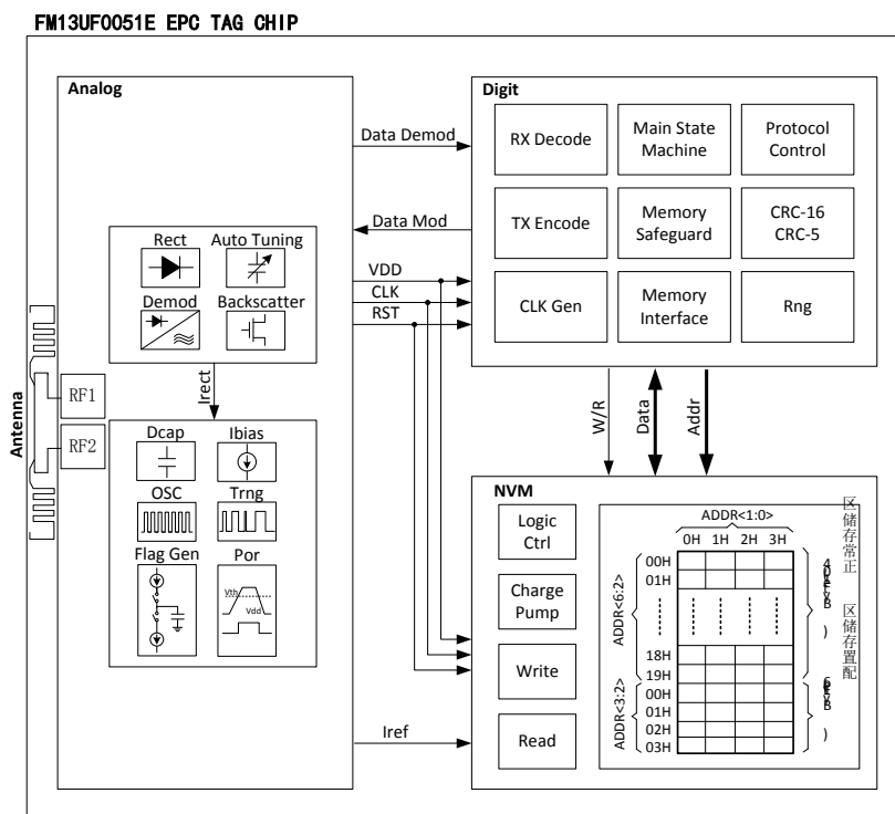
图 2-1 结构框图
