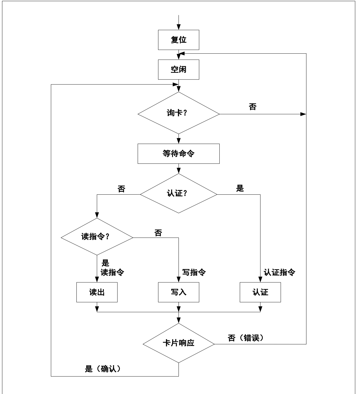
图 4-1 FM11RF005M 卡状态转换图
