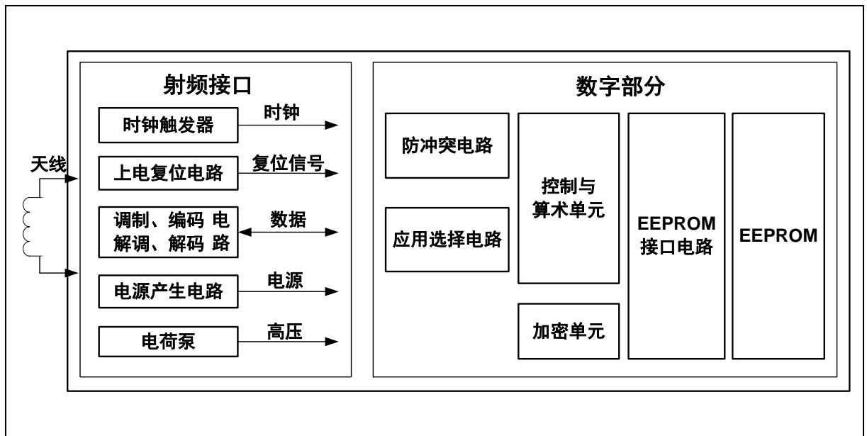
图 2-1 FM11RF005M 结构框图
