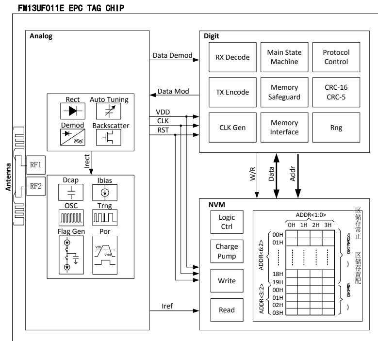
图 2-1 结构框图
