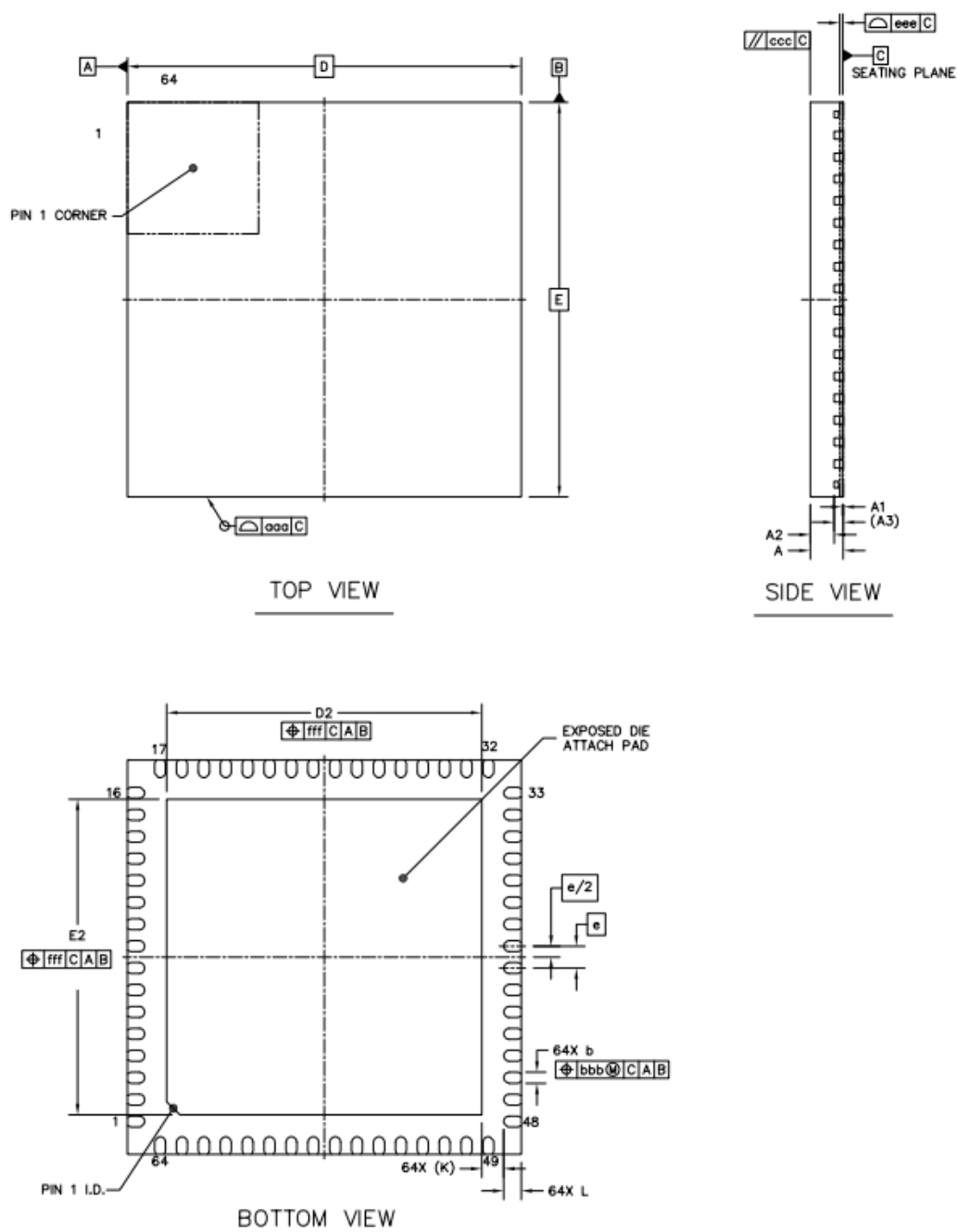
图 6-1 RD1616G 芯片封装顶视和尺寸图
