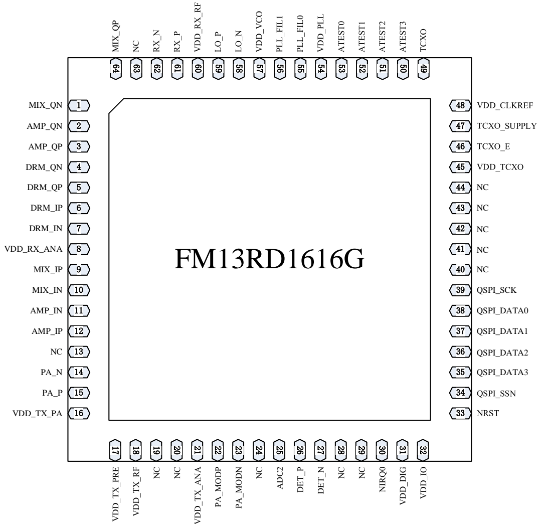
图 2-2 RD1616G 读写器管脚示意图
